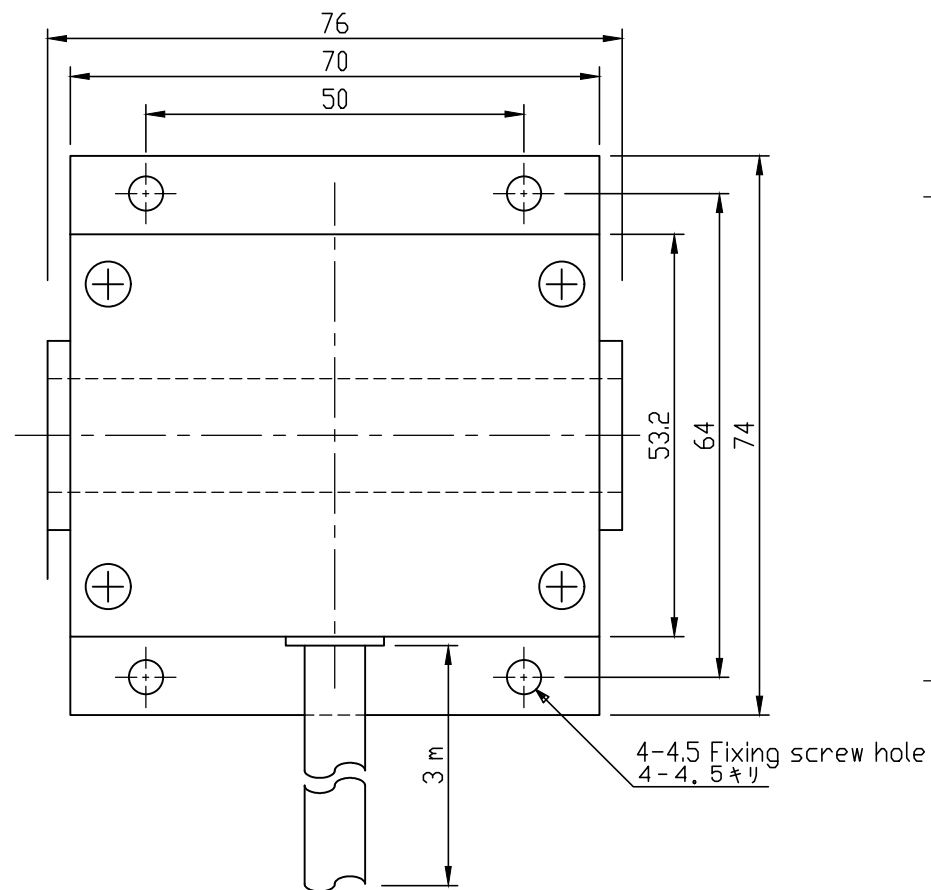
取り付けネジ寸法図 Fixing screw hole dimension
