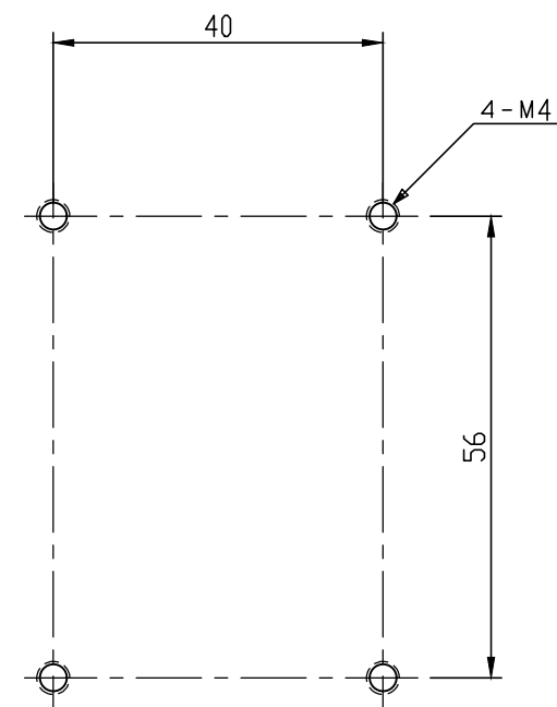
取り付けネジ寸法図 Fixing screw hole dimension
