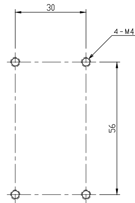
取り付けネジ寸法図 Fixing screw hole dimension
