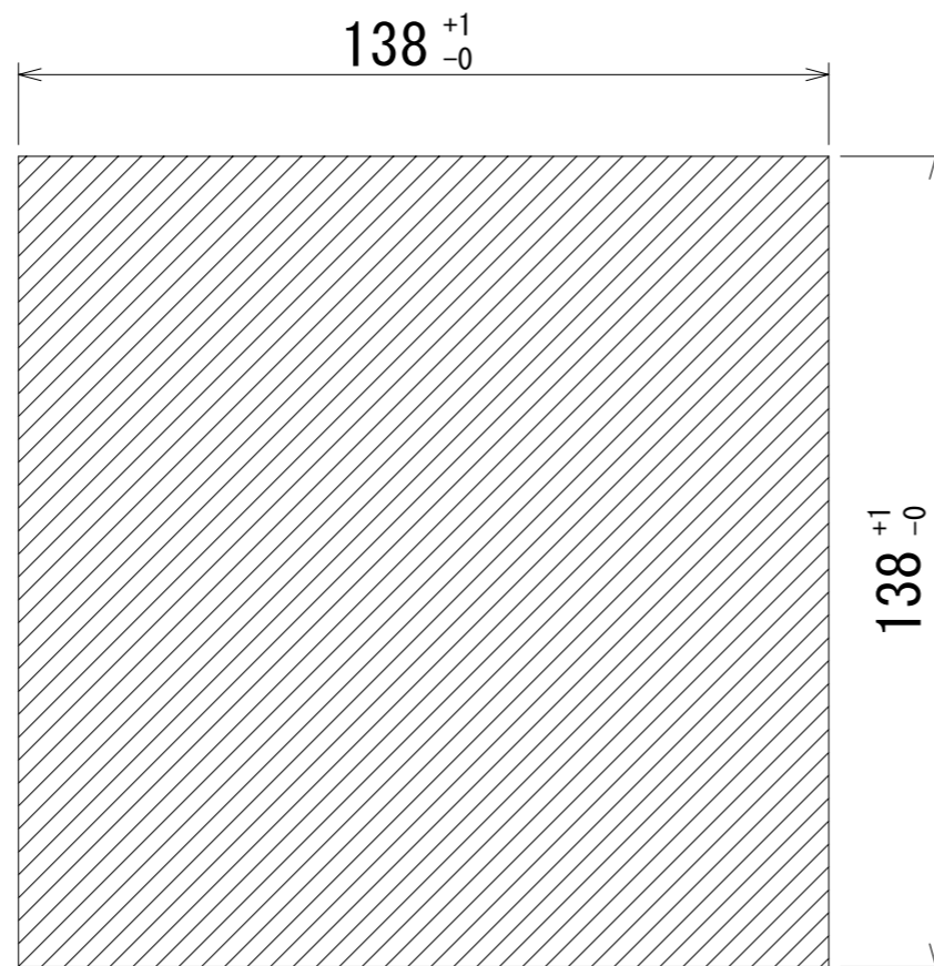
パネルカット寸法 Panel Cut Dimention
