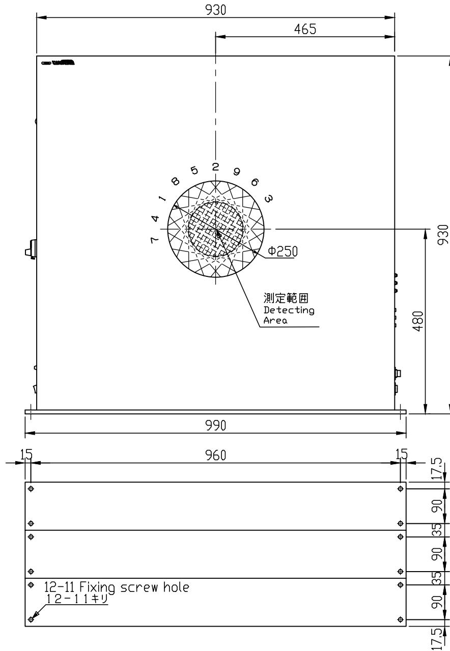
TM-7009 外形図 Outline Drawing
