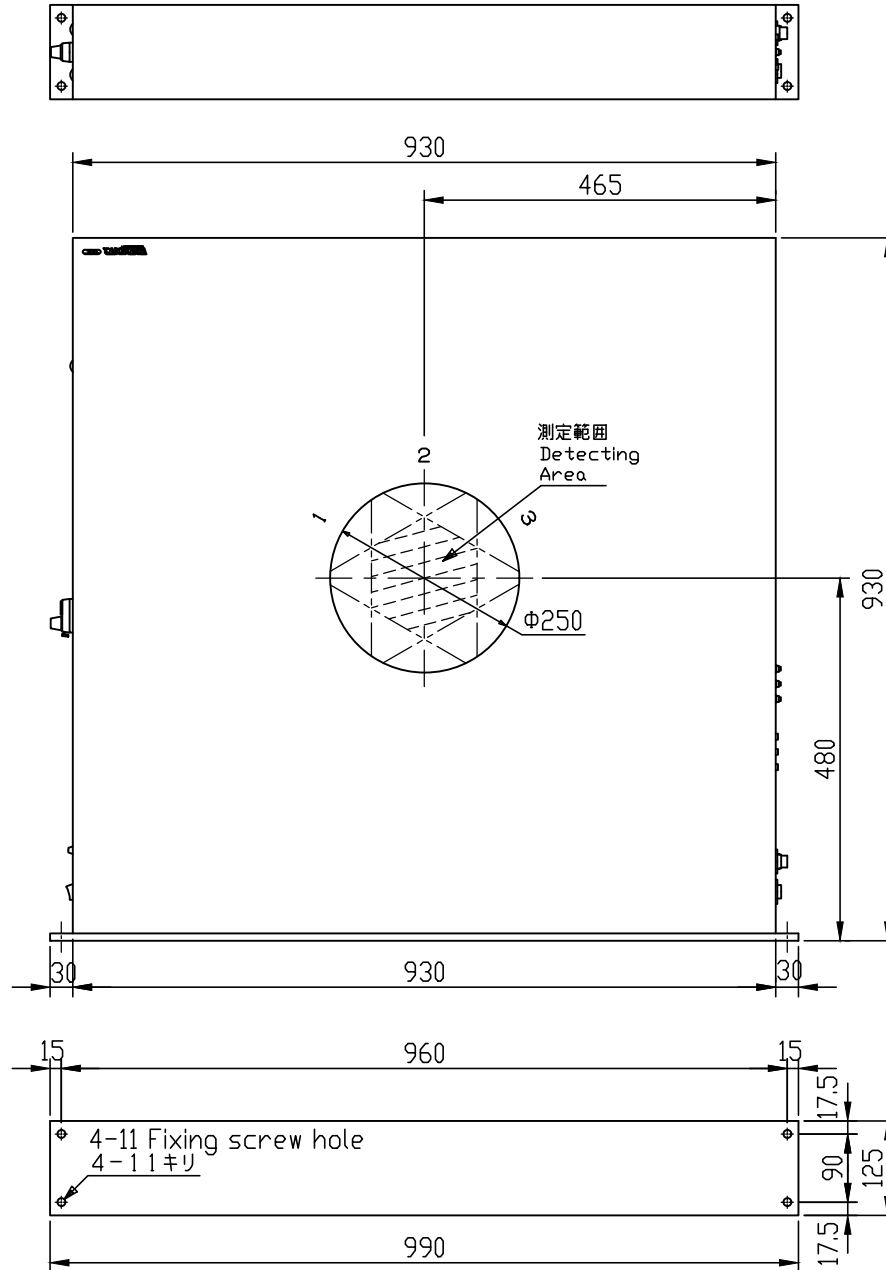
TM-7003A 外形図 OutLine Drawing
