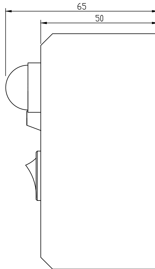
PW-02 外形图 Outline Drawing
