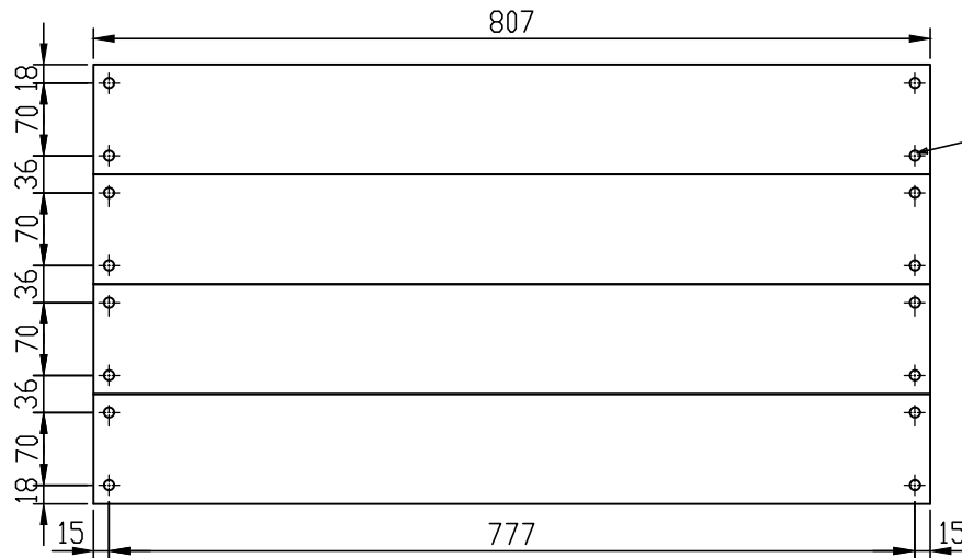
TM-4016 外形図 Outline Drawing
