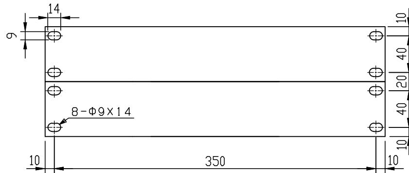
TM-3008W 外形図
