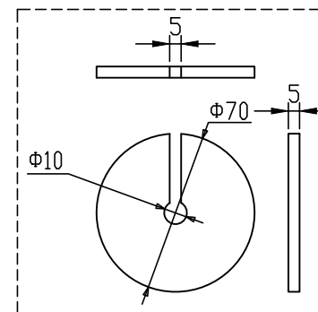
センターガイド Center Guide
