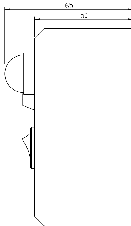
PW-01 外形图 Outline Drawing
