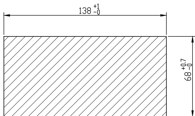
パネルカット寸法 Panel Cut Dimensions
