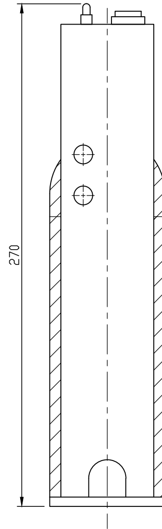
MAC-01 外形図 OutLine Drawing
