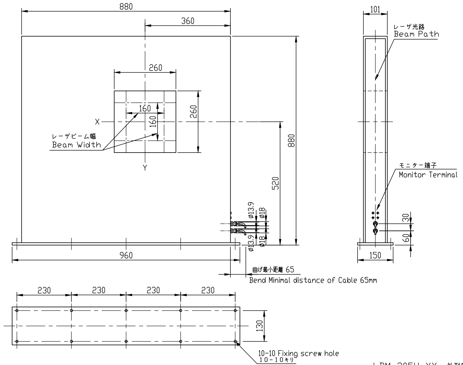
LDM-305H-XY 外形図
