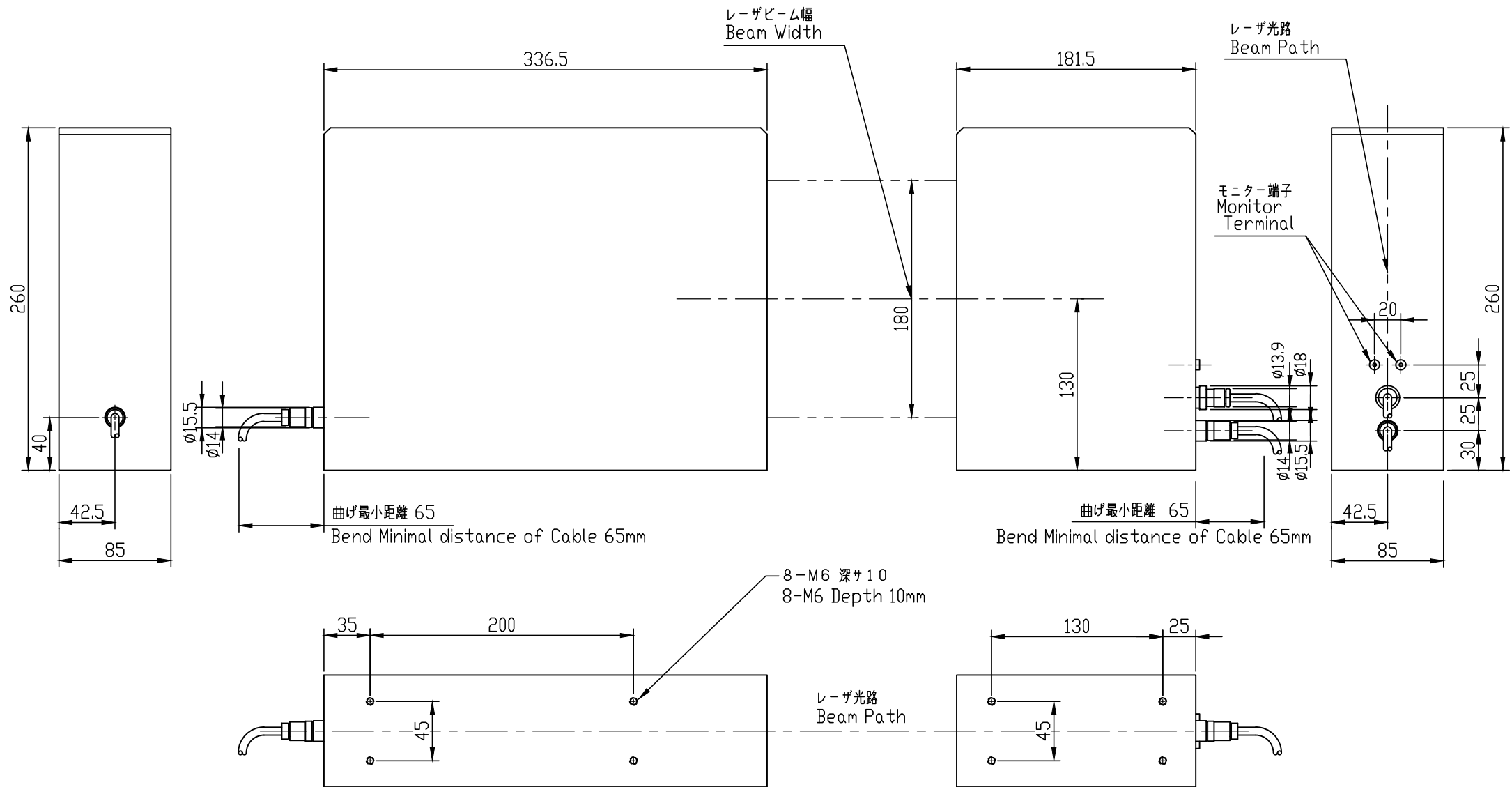
LDM-305H-SP 外形図
