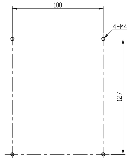
取り付けネジ寸法図 Fixing screw hole dimension
