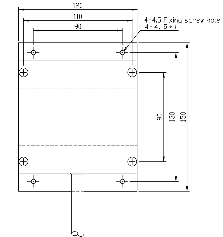
IDS-60 外形図 Outline Drawing
