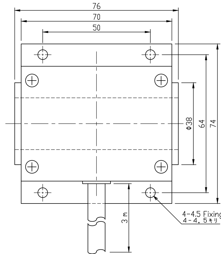
取り付けネジ寸法図 Fixing screw hole dimension
