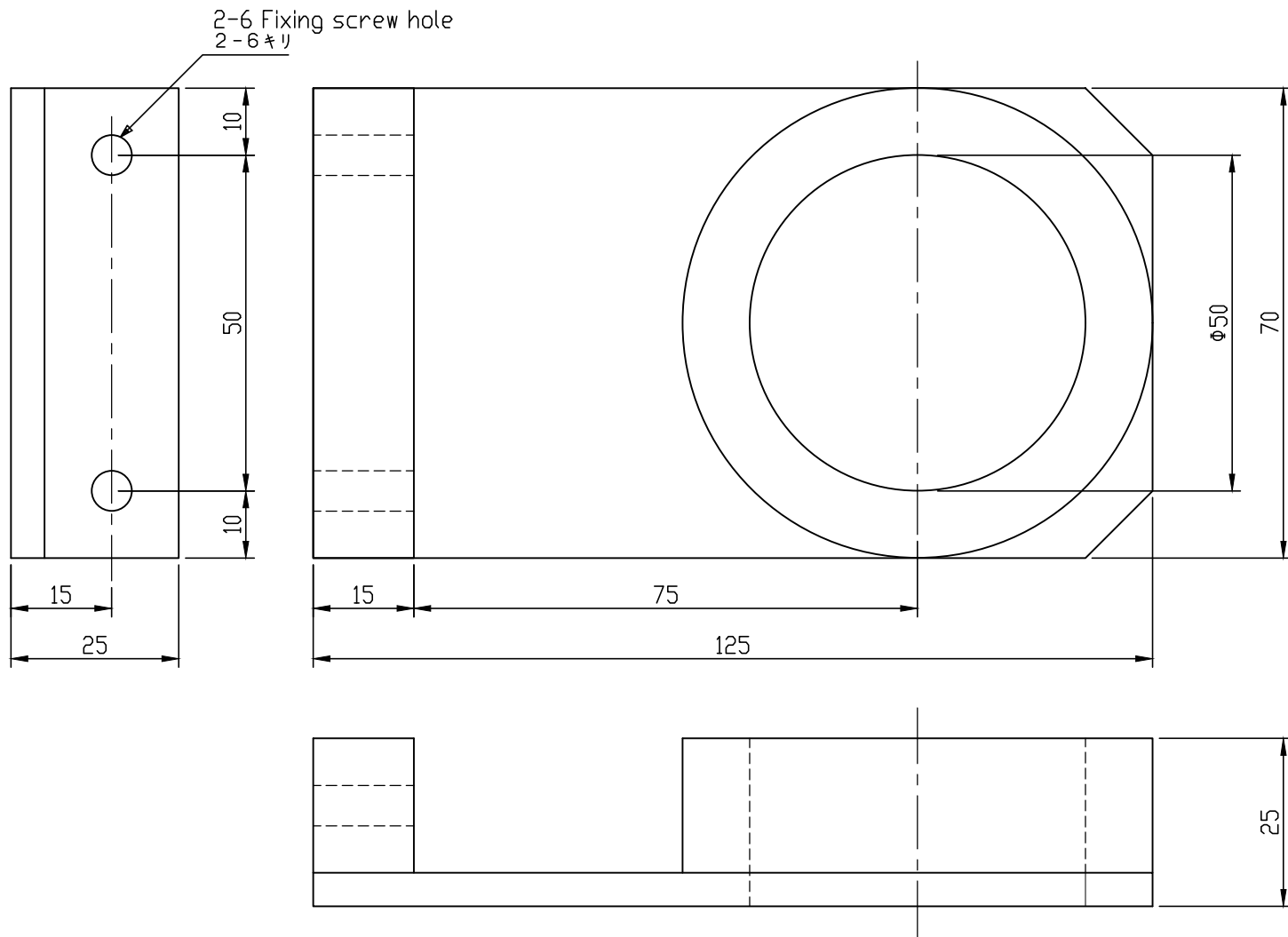
ID-50 外形図 Outline Drawing
