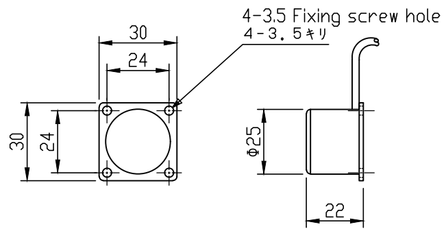
検出部 Sensor
