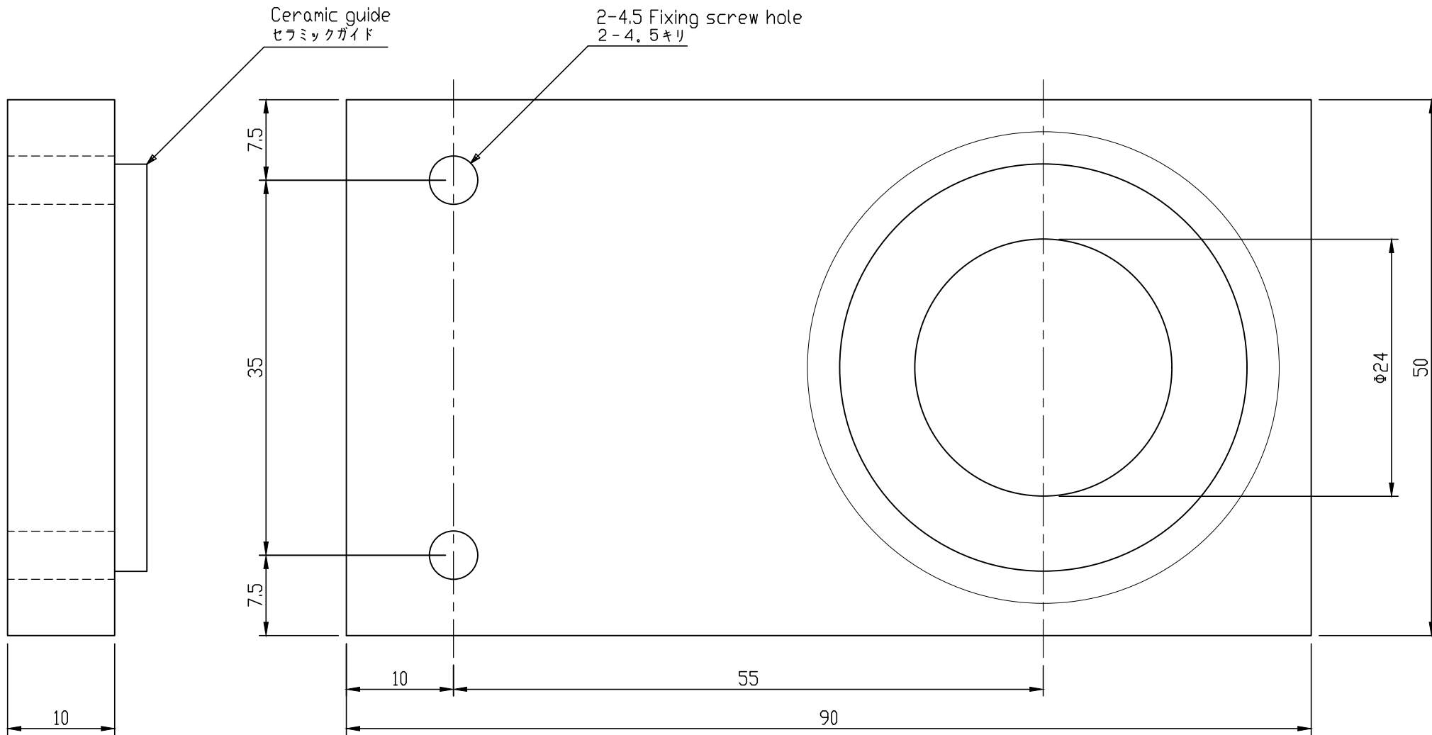
ID-30 外形図 Outline Drawing
