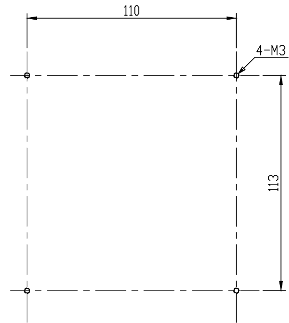
取り付けネジ寸法図 Fixing screw hole dimension
