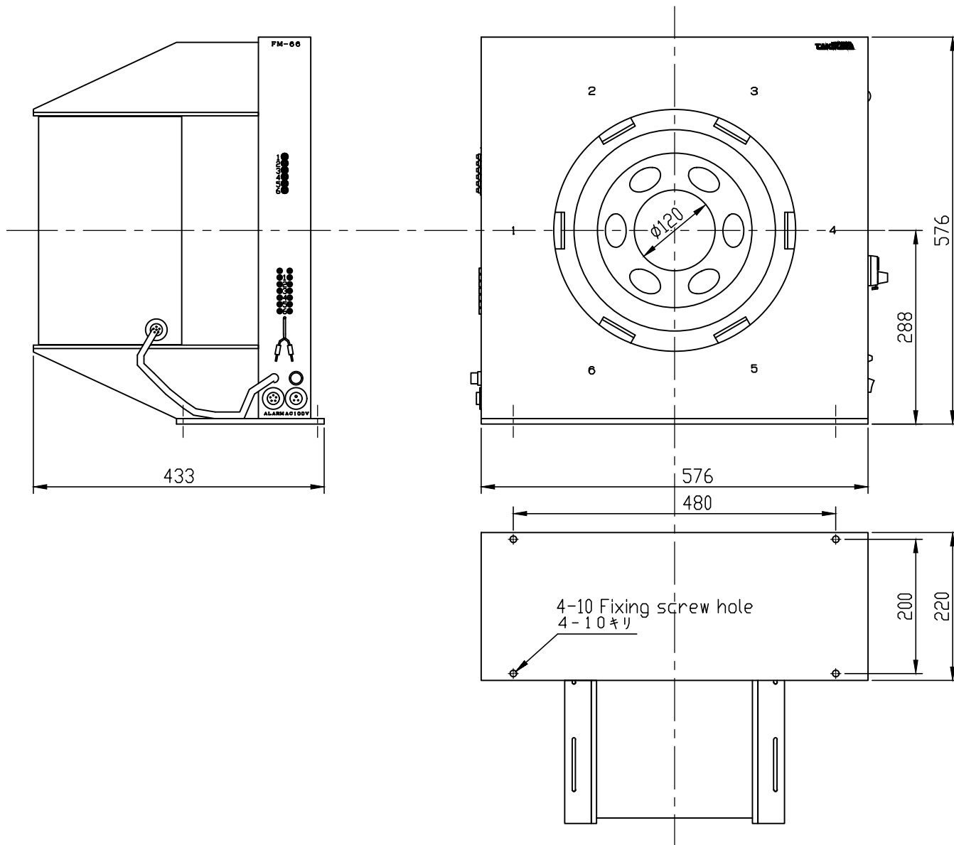
FM-66L 外形図 Outline Drawing
