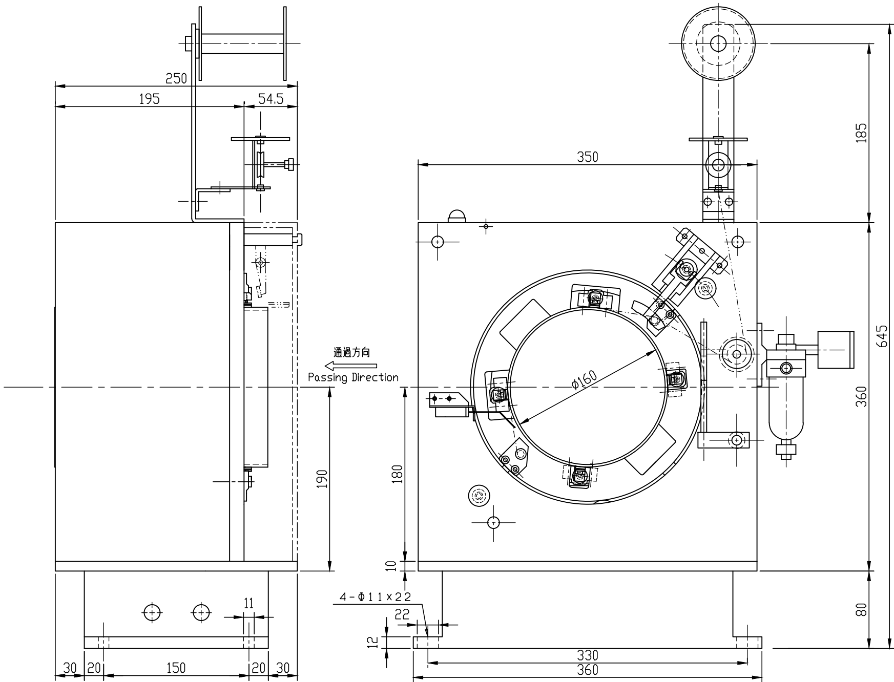
EMAC-160 外形圖 OutLine Drawing
