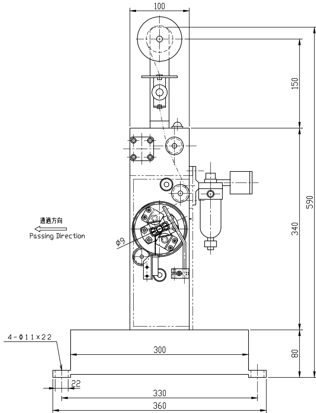
EMAC-009 外形圖 OutLine Drawing
