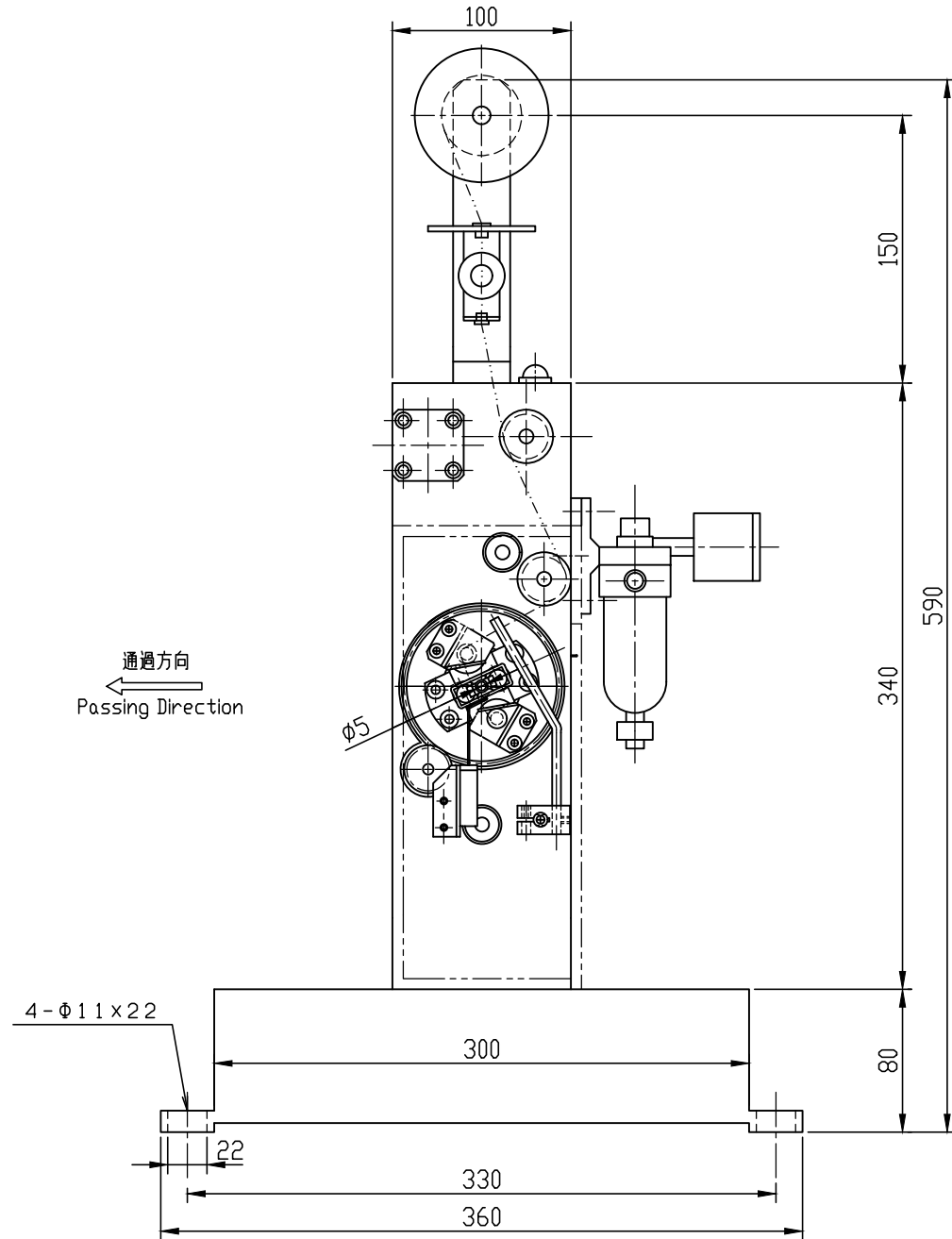
EMAC-005 外形圖 OutLine Drawing
