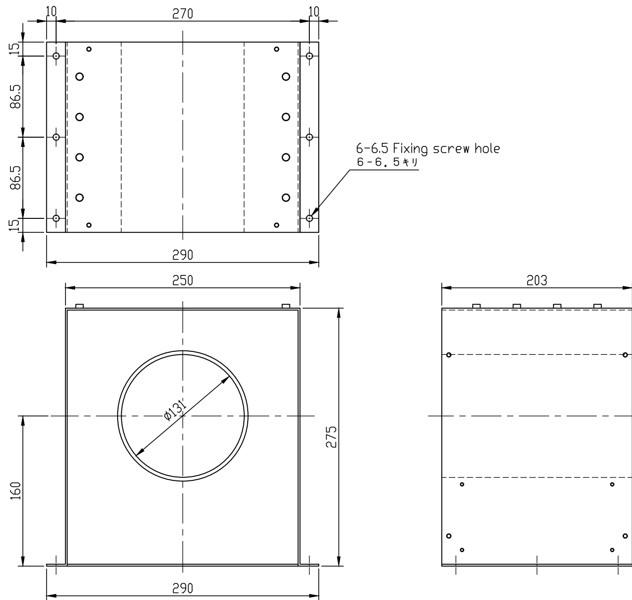
EM-125 外形図 Outline Drawing
