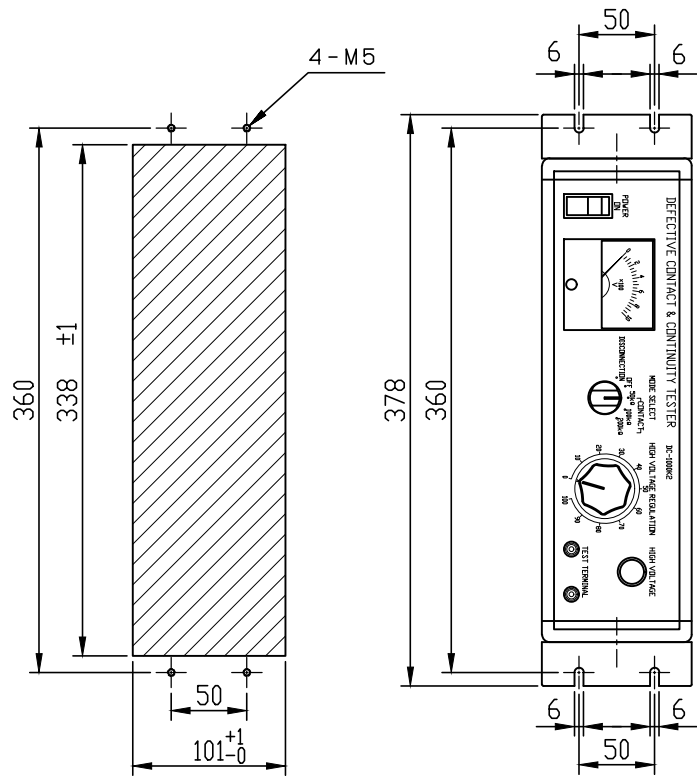
パネルカット寸法 Panel Cut Dimensions
