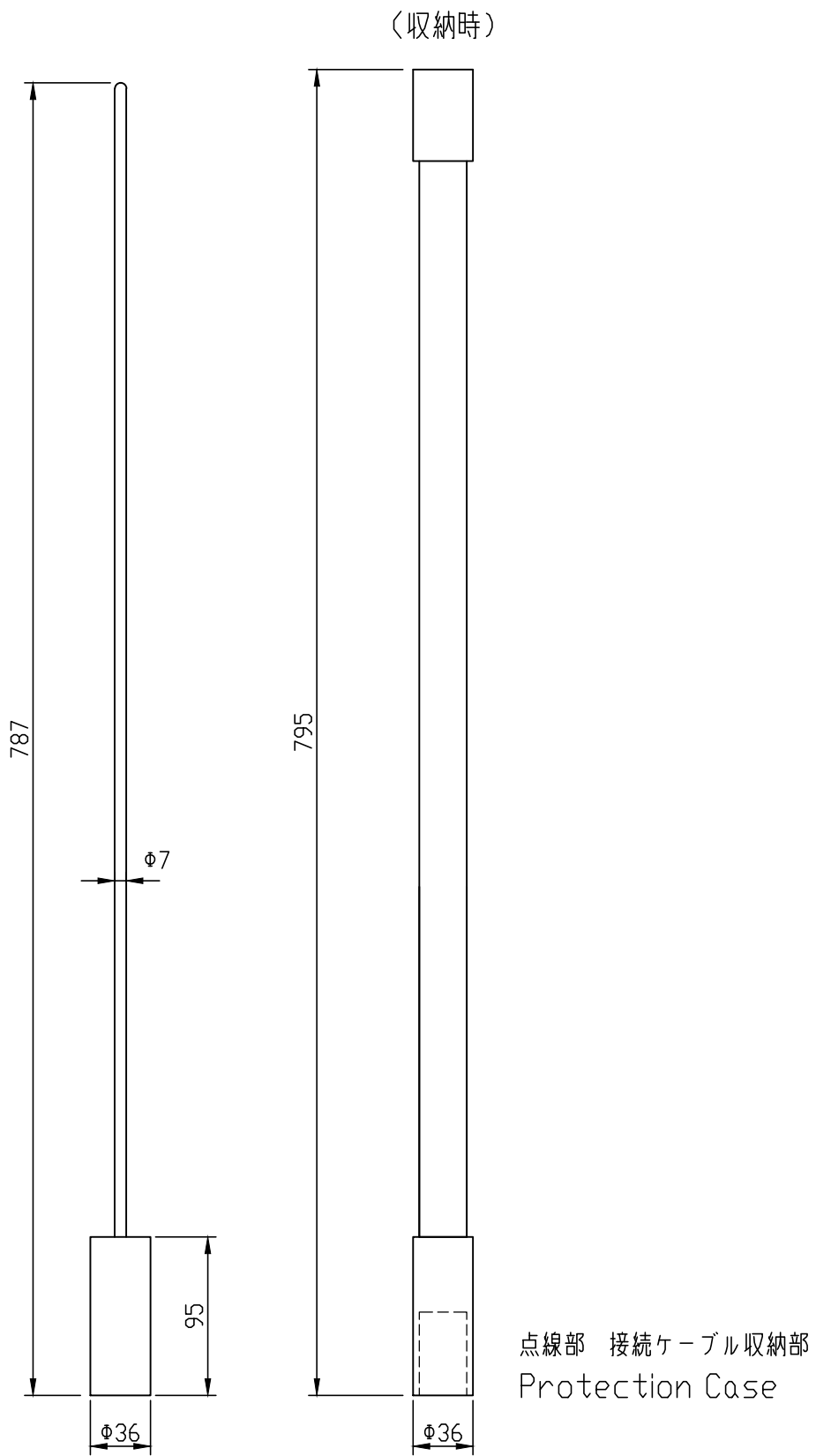
CPR-15 外形図 Outline Drawing
