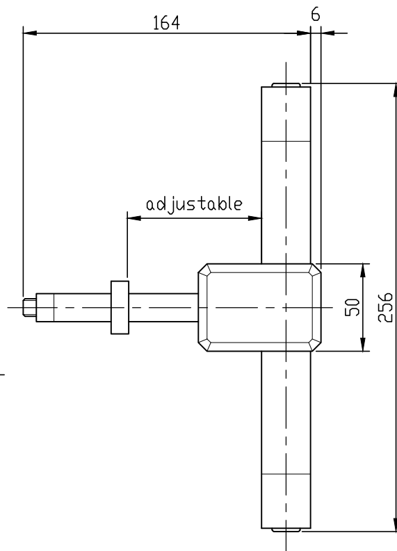
CP-05B 外形图 Outline Drawing
