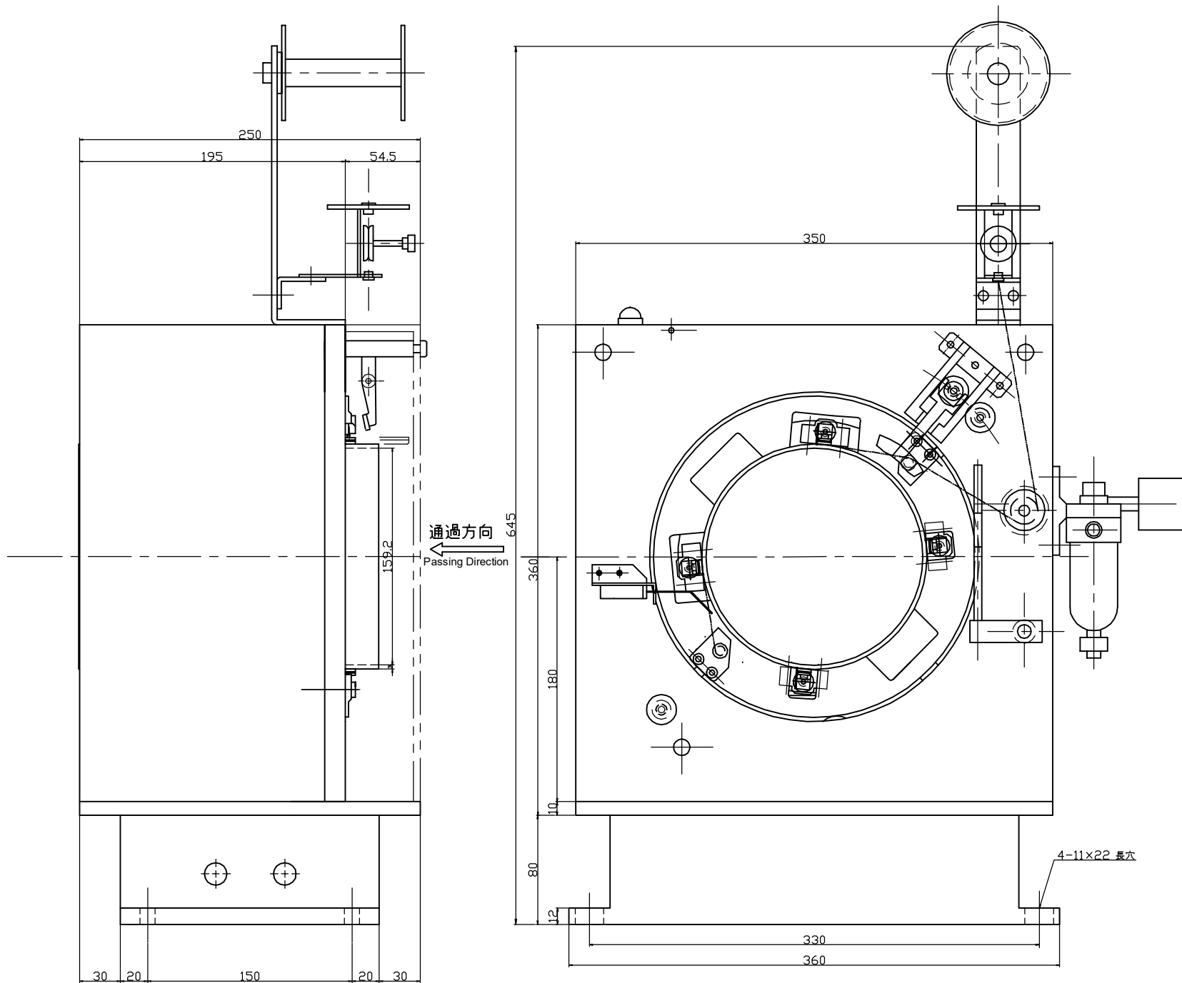
EMAC-160 外觀圖 OutLine Drawing
