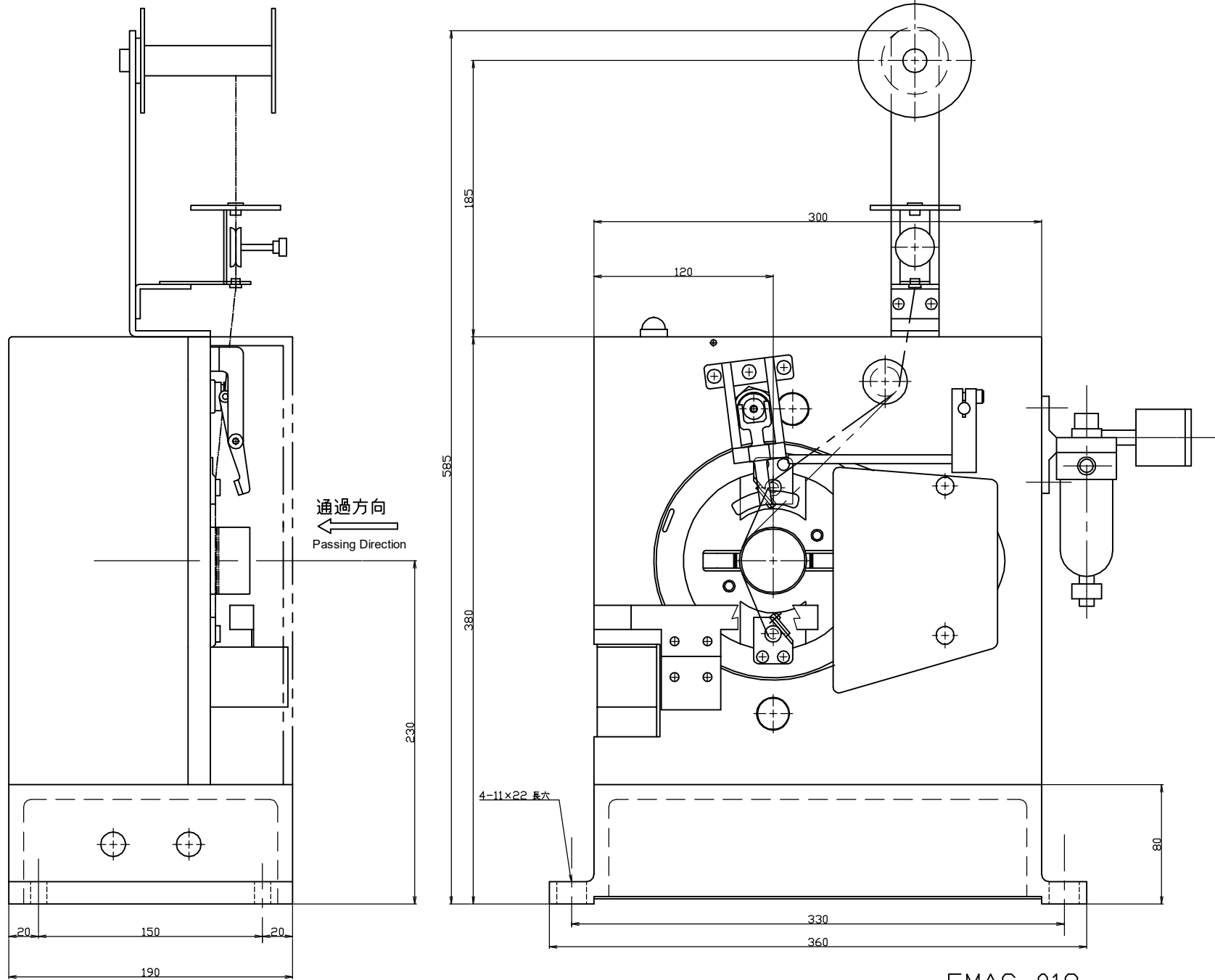
EMAC-019 外觀圖 Outline Drawing
