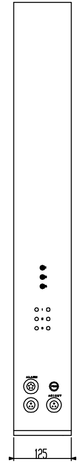
TM-7003 外形図 Outline Drawing
