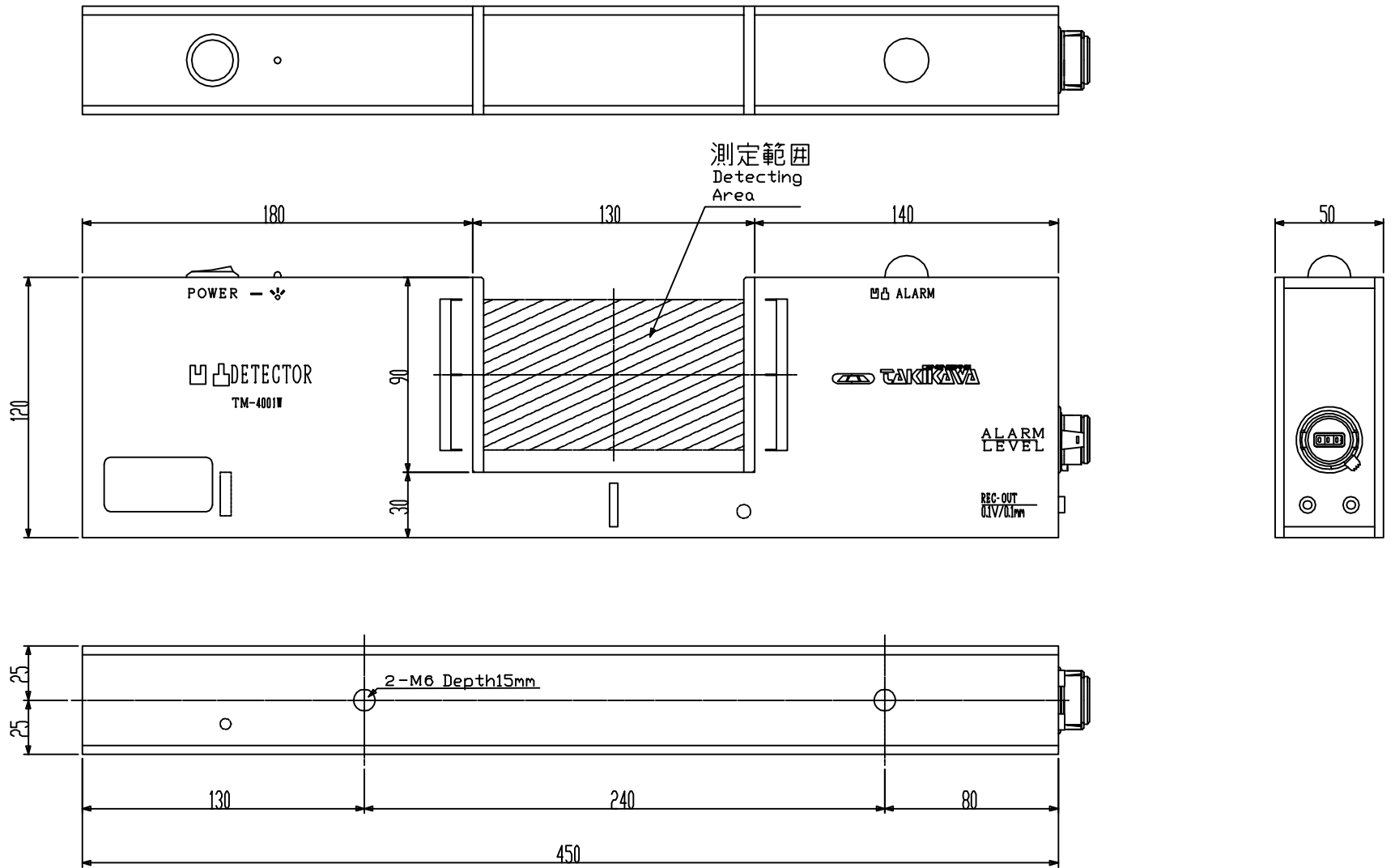
TM- 4001(W) 外形図 OutLine Drawing
