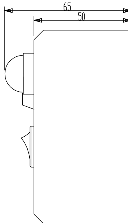
PW-01 外形図 OutLine Drawing
