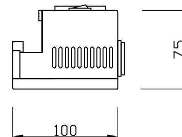
RMR-01 外觀図 OutLine Drawing
