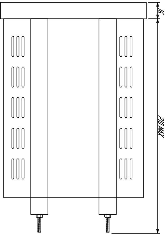
TMS-01 外形図 Outline Drawing
